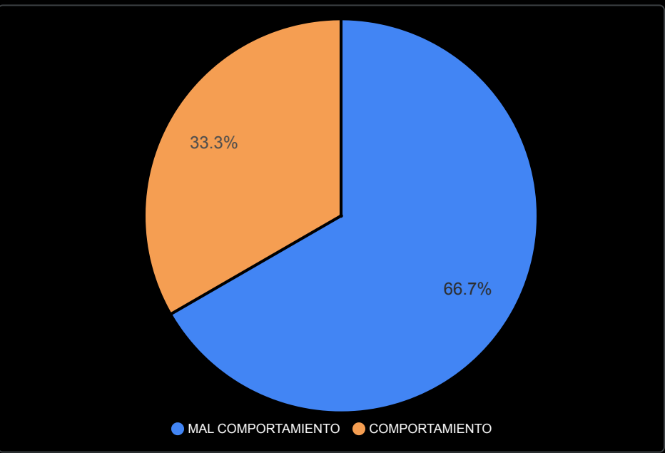
DISTRIBUCION DE LAS OBSERVACIONES
