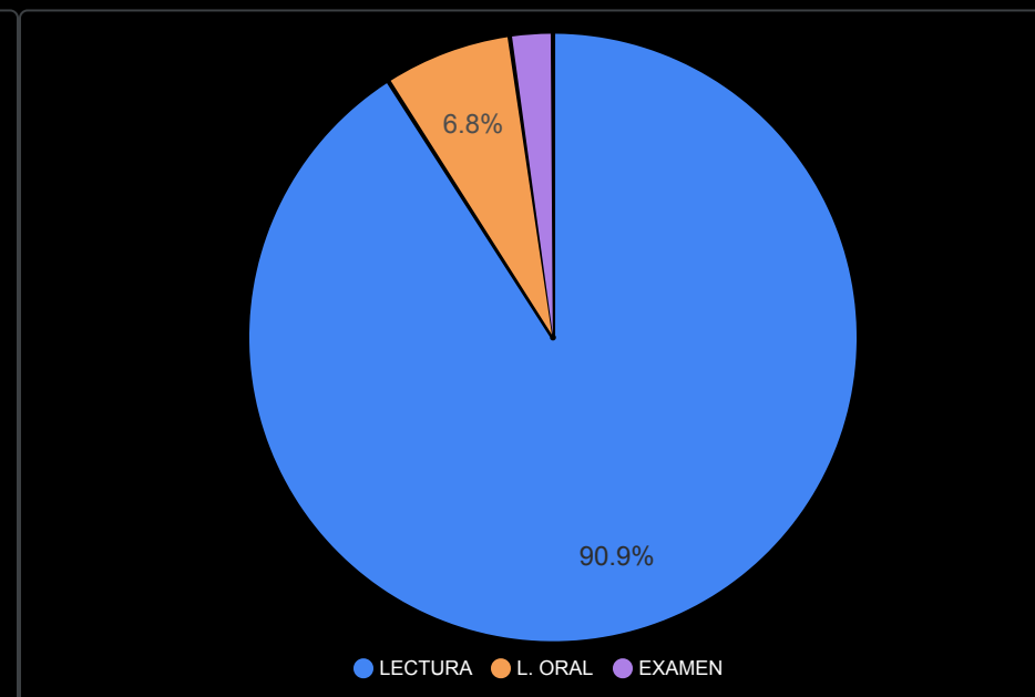
APORTE NOTA x TIPO DE EVALUACION
