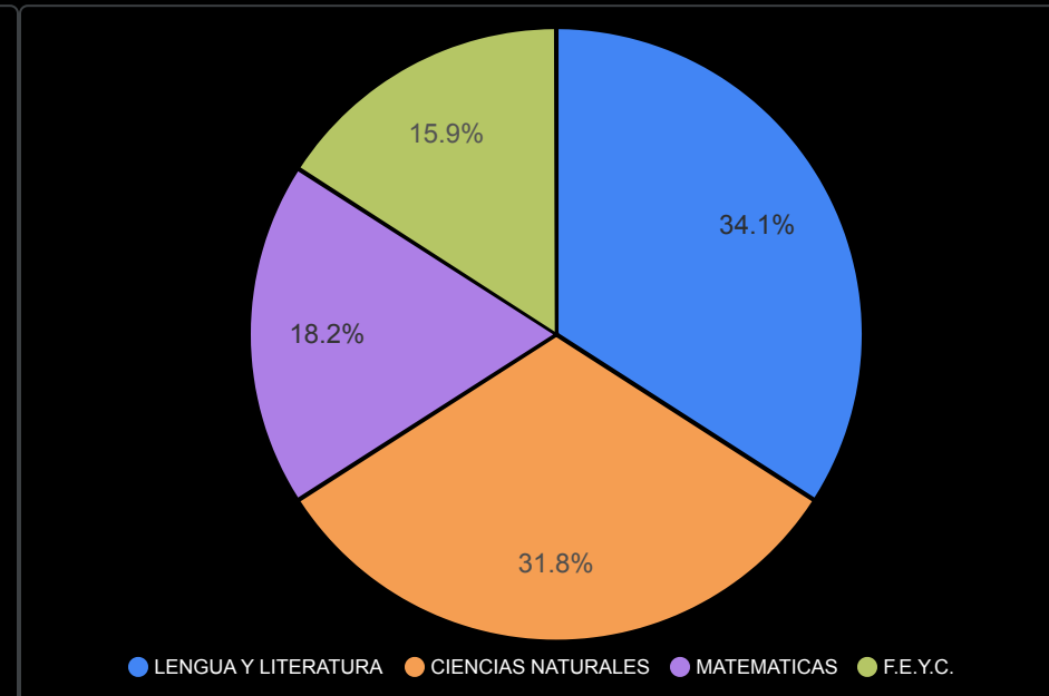
APORTE NOTA x TIPO DE EVALUACION y MATERIA
