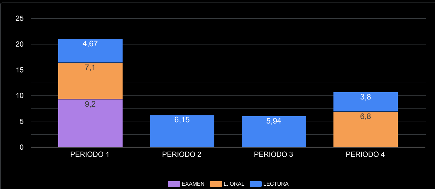
PROMEDIO NOTA x TIPO DE EVALUACION
