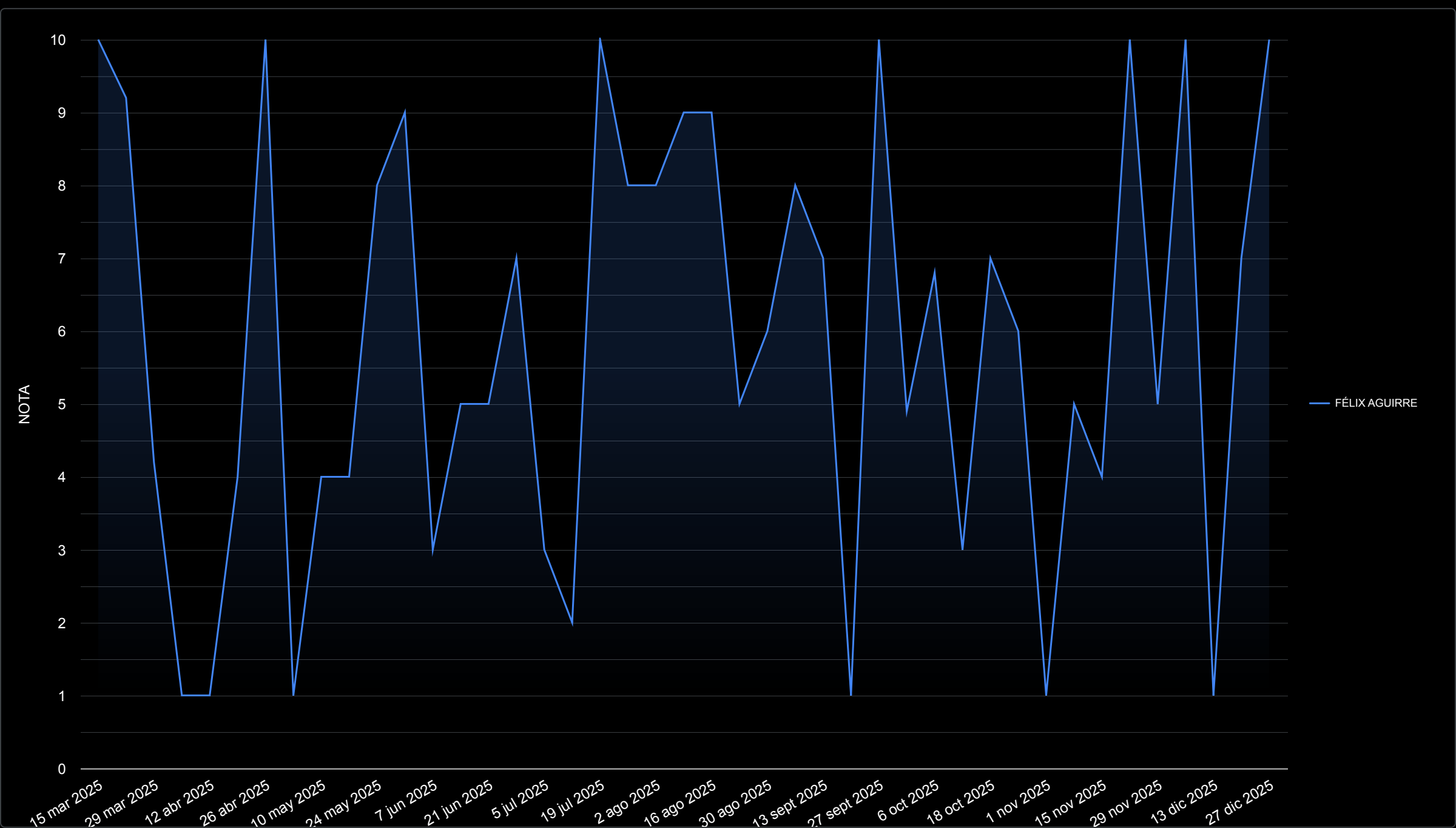
Evolucion Nota Anual x Alumno
