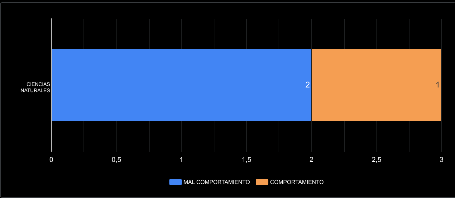
CANTIDAD DE OBSERVACIONES X MATERIA X PERIODO
