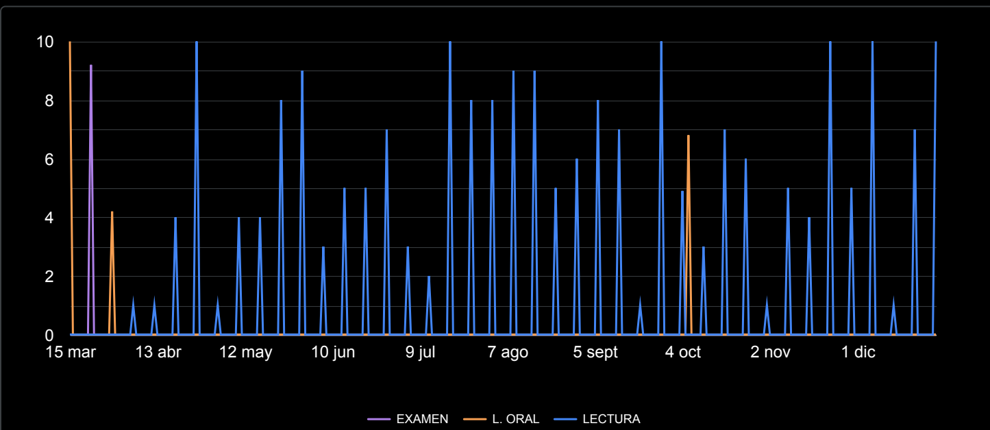
PROMEDIO NOTA x TIPO DE EVALUACION y MATERIA
